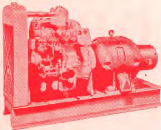
Equipo generador eléctrico Diesel, enfriado por agua, con una salida de 15 kv. Uno de los muchos generadores de energía sistema Diesel con salidas de 3 a 90 kv. Se adaptan a lugares donde se necesite mucha energía . . . fábricas, edificios públicos, aldeas o poblaciones.
